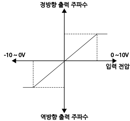
[양방향 전압 입력 및 출력 주파수]
