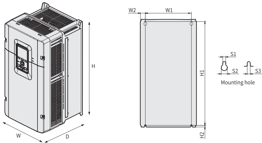
외형 치수(200V급 22kW / 400V급 30~37kW)
