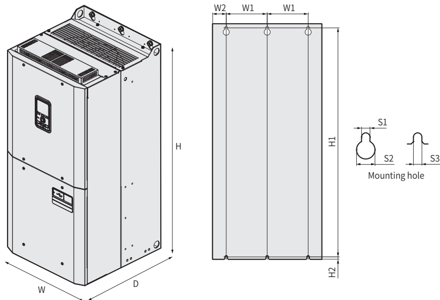
외형 치수(400V급 185 ~ 220kW)
