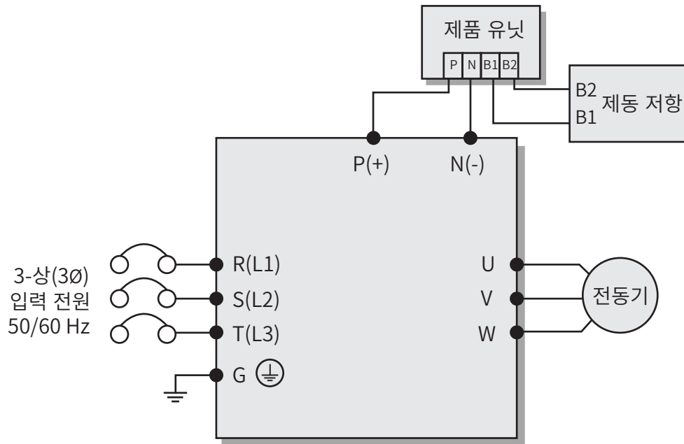
[제동 유닛 및 제동 저항 기본 결선도]
