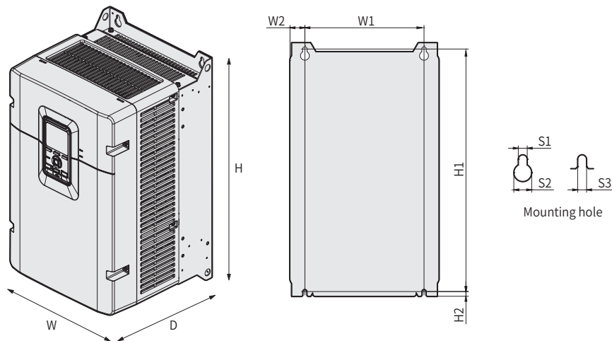
외형 치수(200V급 30kW / 400V급 45kW)
