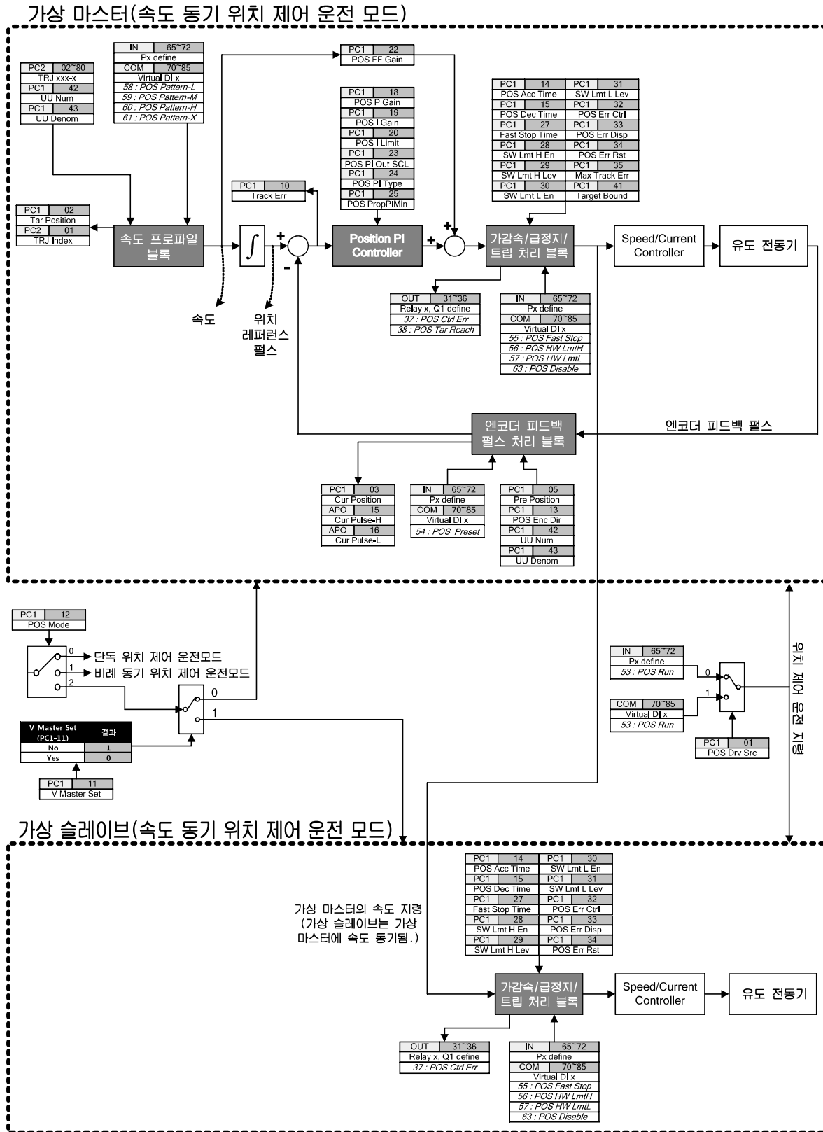
A.2.2.1 속도 동기 위치 제어 운전 모드의 전체 블록도
