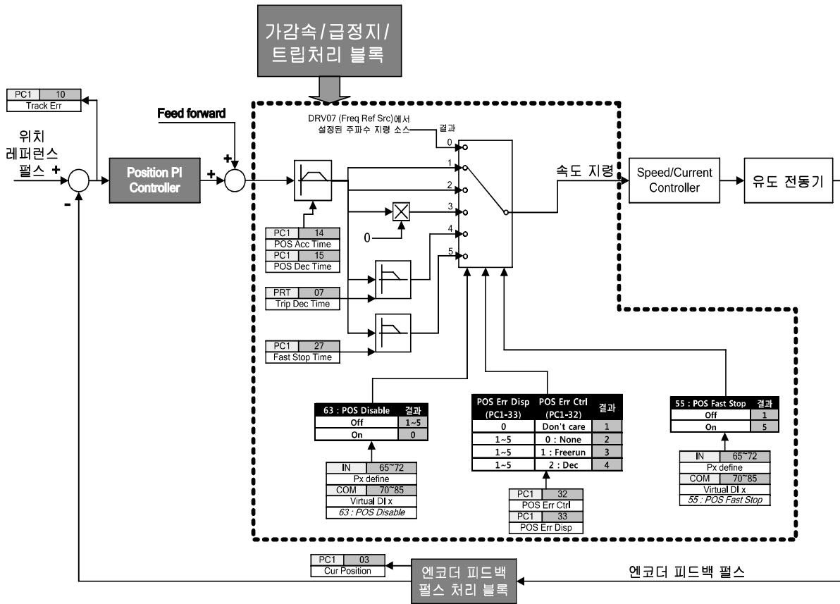
그림 3.5 예외 처리 블록도
