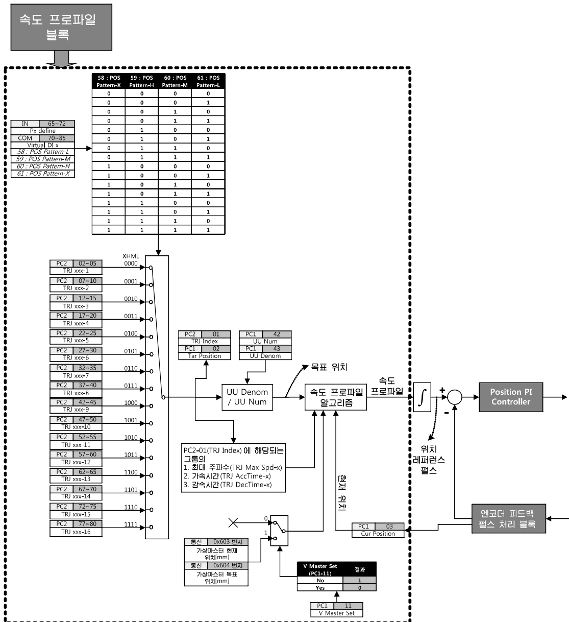
그림 A.3 위치 경로 선택 블록
