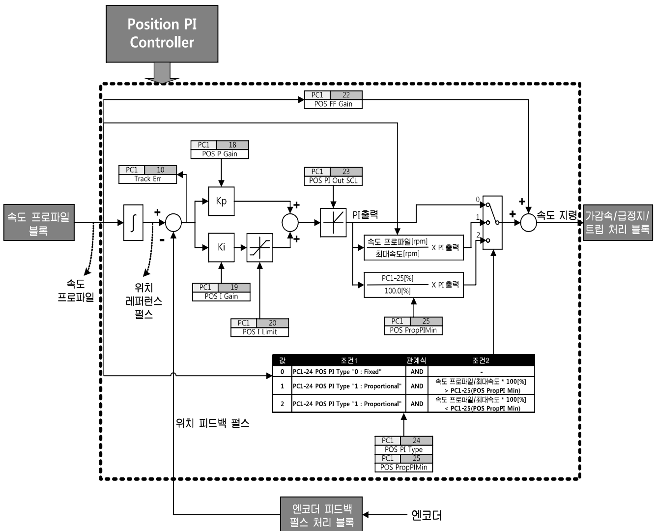
그림 3.4 Position PI Controller 블록도
