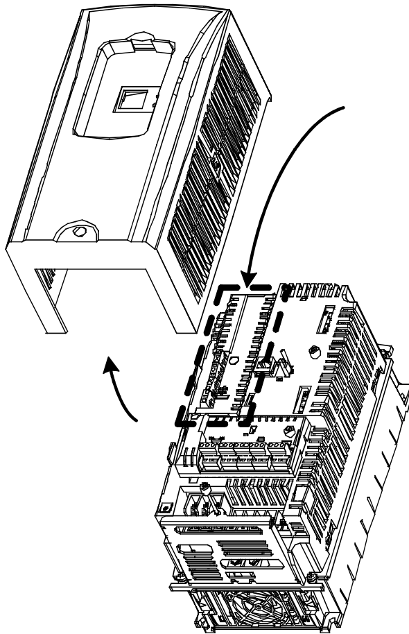
그림 2.1 iS7 위치 제어 전용 엔코더 옵션 장착
