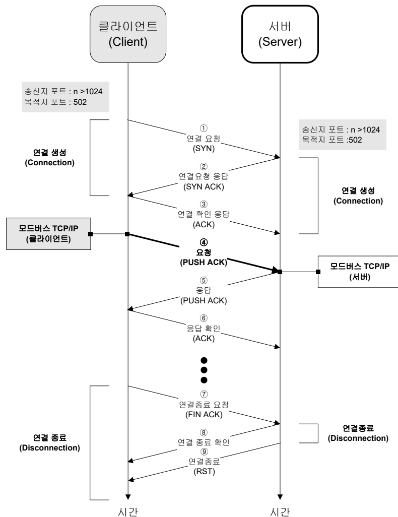
[그림 7-31] TCP XGT 클라이언트 채널 설정
