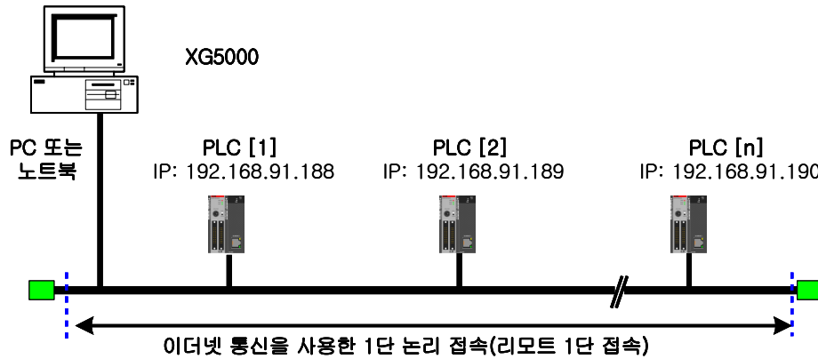
[그림 9-6] PC 를 통한 리모트 1 단 접속 시스템
