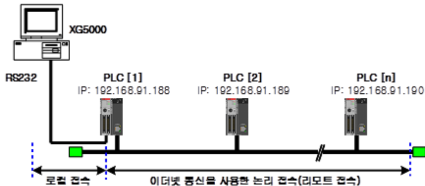
[그림 9-1] 리모트 접속 개요
