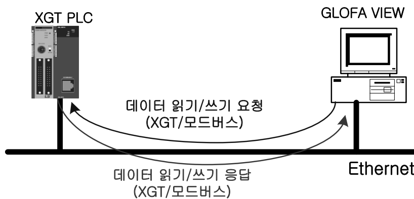
[그림 7-7] 이더넷(서버) 드라이버 사용 예
