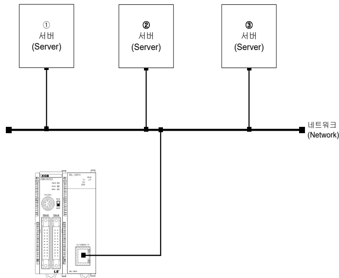
[그림 7-2] 클라이언트/서버 시스템 구성
