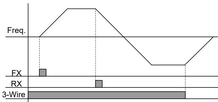
[3-와이어 운전]
