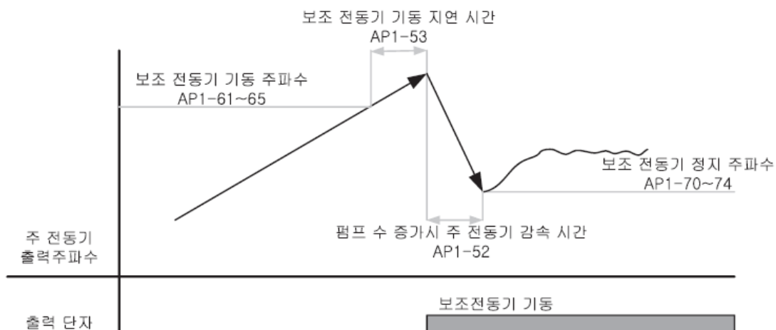
부하 증가에 의한 보조 전동기 기동 시퀀스
