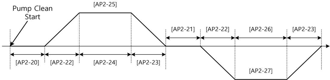
<펌프 클린 기본 운전>
