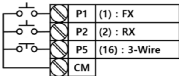
[3-와이어 운전 시 단자 설정]
