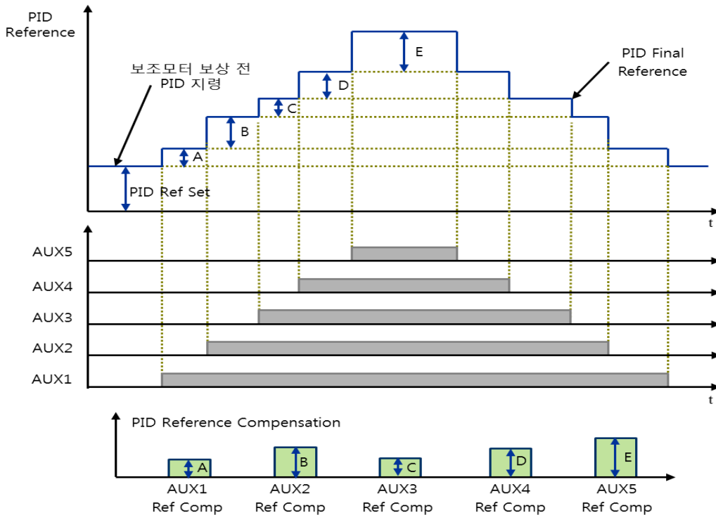
< 보조 모터 PID 보상 기능 >
